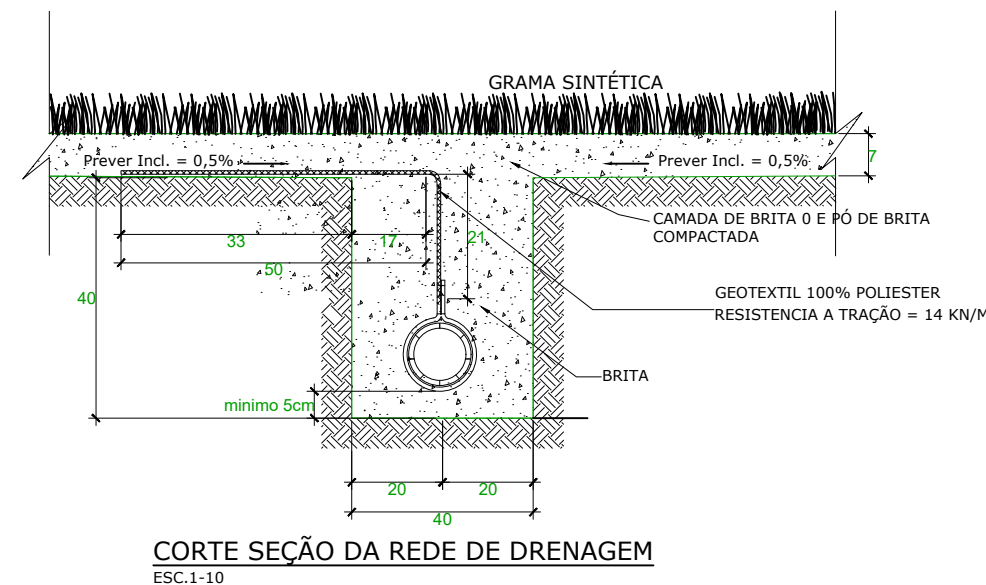
1 CORTE - SEÇÃO DO DRENO SEM ESCALA
