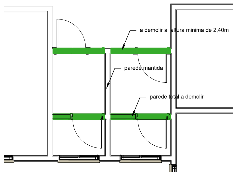
4 DEMOLIÇÕES - WC's 1:50
