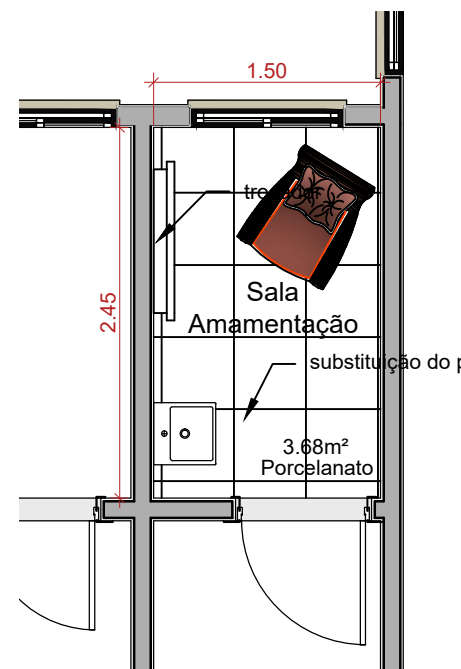
5 PLANTA BAIXA 1:50
