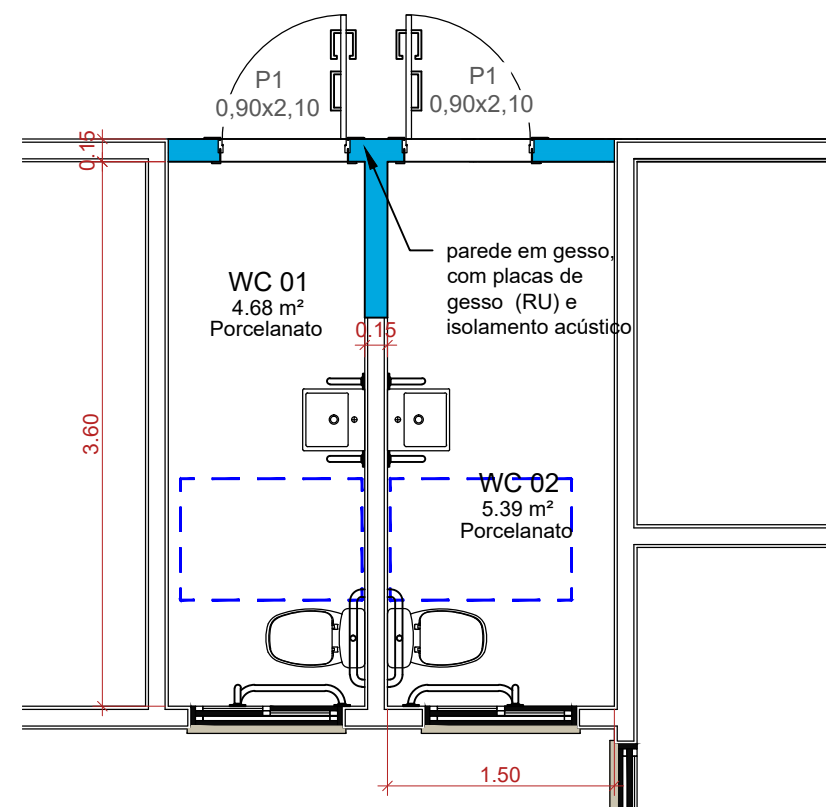
3 NOVAS INSTALAÇÕES - WC's 1:50
