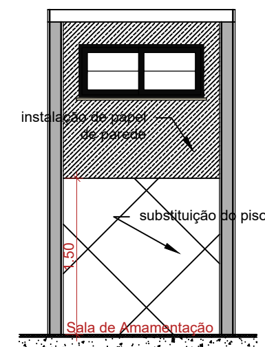
1 CORTE - S. AMAM. 1:50
