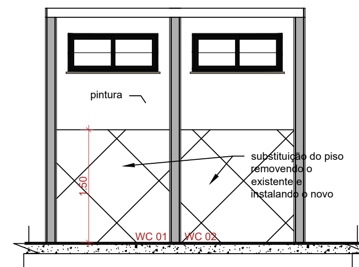
2 CORTE - WC's 1:50
