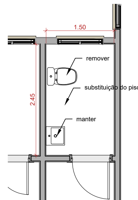
6 REMOÇÃO - S. AMAM. 1:50
